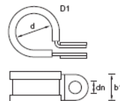
Colliers de fixation SQ
